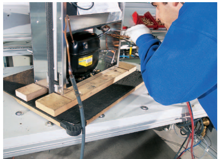
Sistema di montaggio manuale per la produzione di frigoriferi di fino a 75 kg di peso e a 2 m di altezza Sistema de montaje manual para la producción de equipos de refrigeración de hasta 75 kg de peso y 2 m de altura Sistema de montagem manual para a produção de refrigeradores com um peso de até 75 kg e altura de 2 m Pfannerberg GmbH, Hamburg, D Made by Handke Industrietechnik, Hamburg, D
