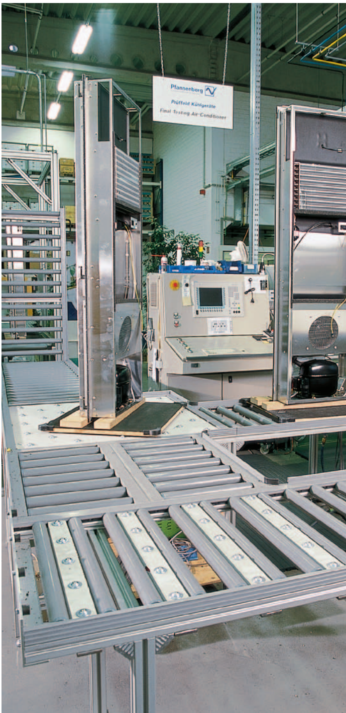
Sistema di montaggio manuale per la produzione di frigoriferi di fino a 75 kg di peso e a 2 m di altezza Sistema de montaje manual para la producción de equipos de refrigeración de hasta 75 kg de peso y 2 m de altura Sistema de montagem manual para a produção de refrigeradores com um peso de até 75 kg e altura de 2 m Pfannerberg GmbH, Hamburg, D Made by Handke Industrietechnik, Hamburg, D
