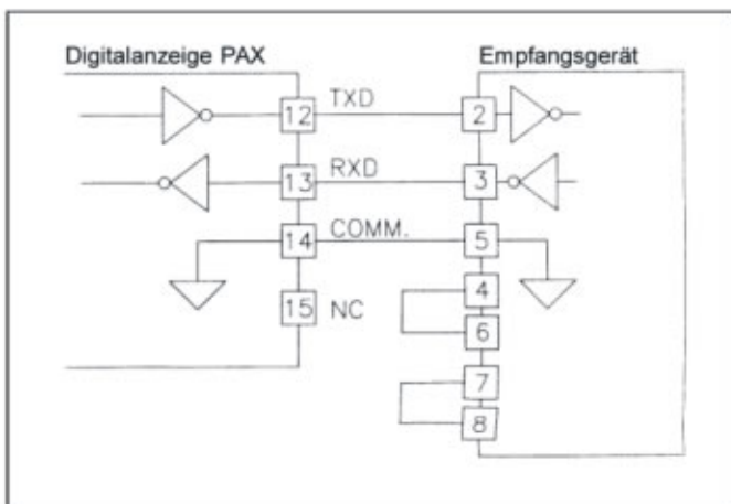
Bild VI: RS232-Schnittstelle
