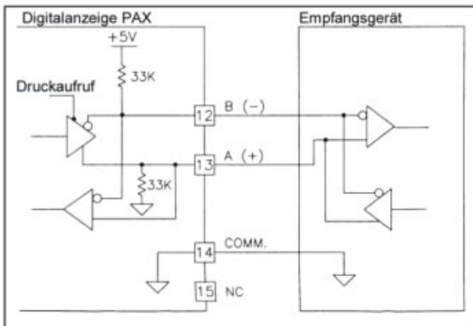
Bild V: RS485-Schnittstelle
