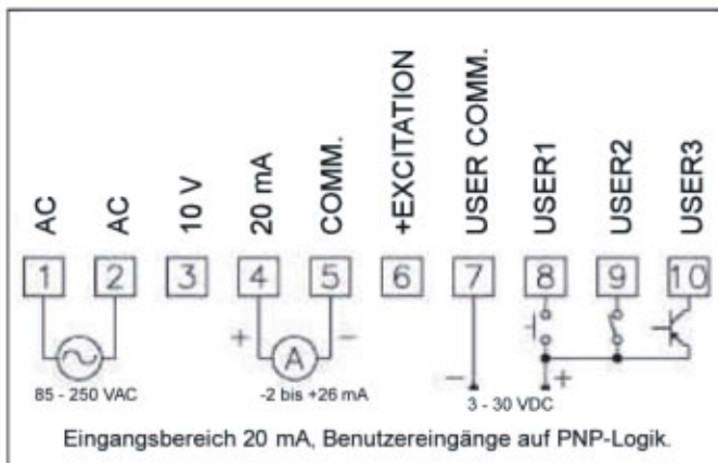
Bild 7.4: Anschlußbeispiel 2: Stromsignal
