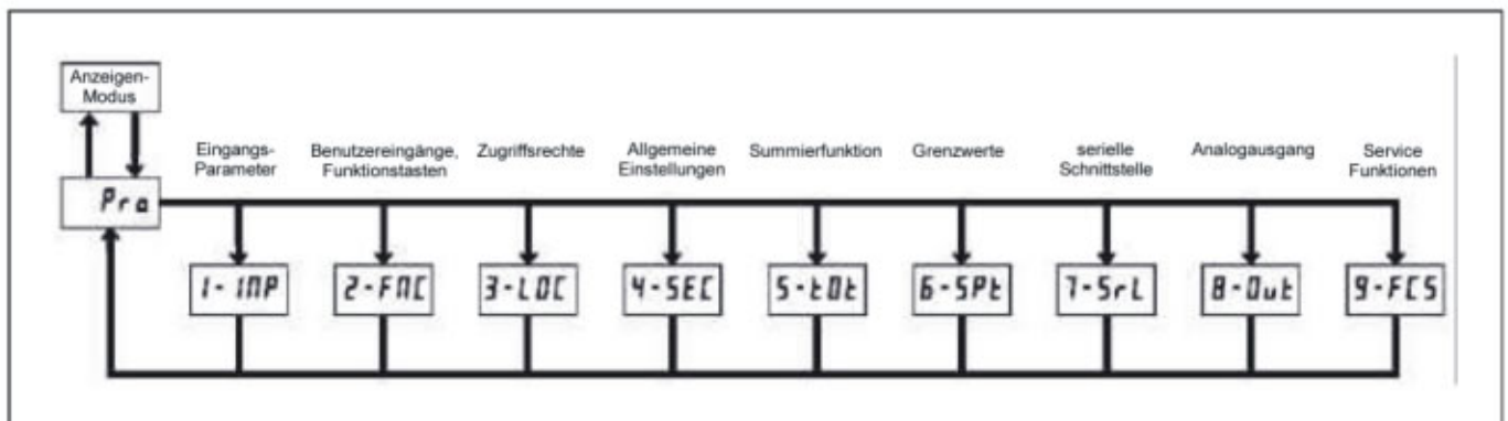
Bild 8.1: Das Programm-Menü
