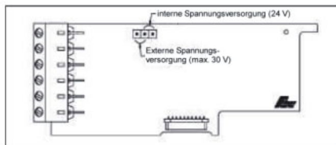
Bild III: Transistorausgangskarte PNP Open-Kollektor
