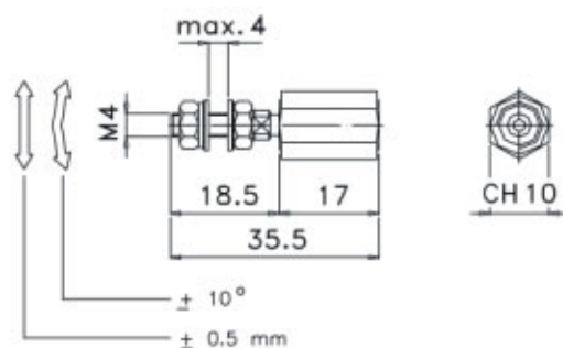
Bearing coupling PKIT020
